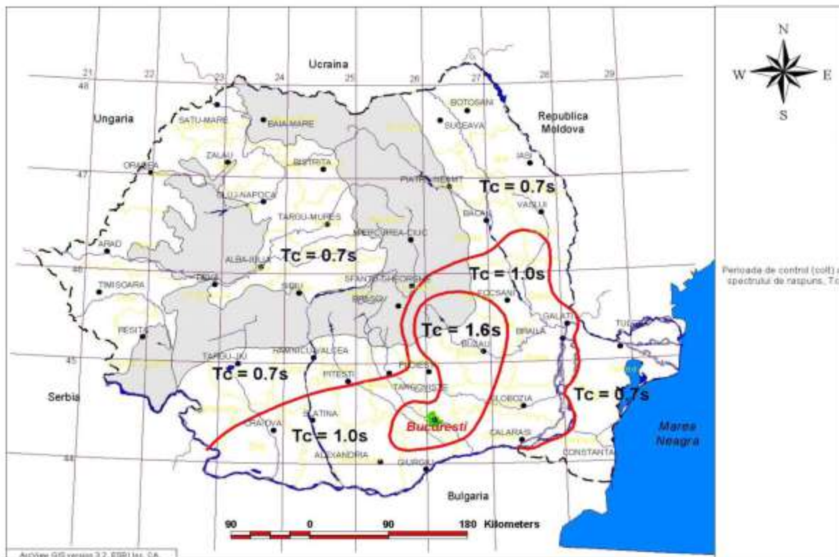
Figura 1 Zonarea teritoriului României în termeni de perioadă de control (colț), T_c a spectrului de răspuns
