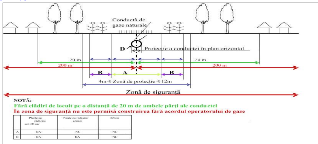
Planul zonelor de protecție și de siguranță în cazul conductelor de alimentare din amonte și de transport gaze naturale
